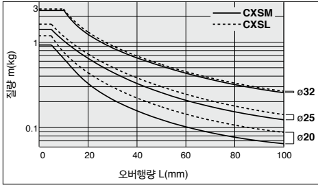
그래프 [8] V=~800mm/s ~30st
