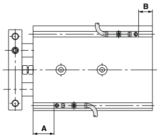
리드선 취출방향 / 안쪽 방향 부착
