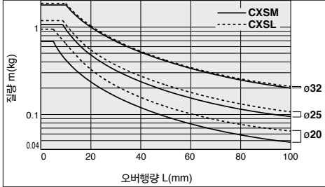
그래프 [10] V=~1000mm/s ~50st
