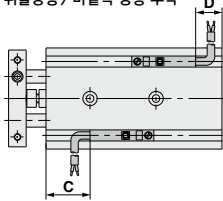
리드선 취출방향 / 바깥쪽 방향 부착
