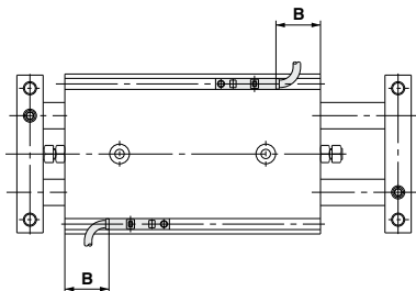
리드선 취출방향 / 바깥쪽 방향 부착
