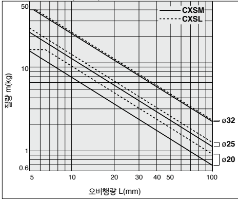
그래프 ③ V=600(mm/s)
