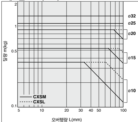
그래프 ⑤ V=600(mm/s)
