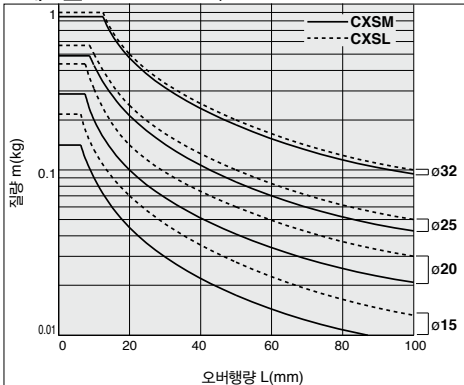
그래프 17 V=400mm/s 초과 ~100st
