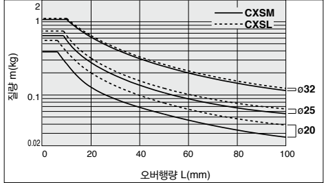
그래프 [11] V=~1000mm/s ~75st
