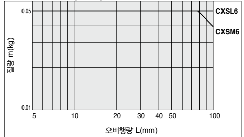
그래프 ② V=300(mm/s)
