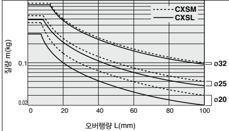
그래프 [12] V=~1000mm/s ~100st
