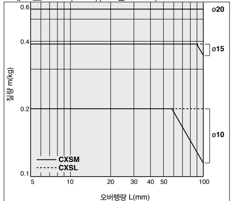
그래프 ⑥ V=700(mm/s)(ø10는 V=800)
