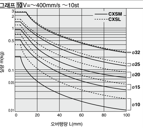
ø10~ø32
