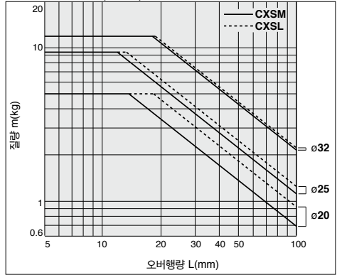
그래프 ④ V=800(mm/s)
