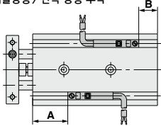
리드선 취출방향 / 안쪽 방향 부착
