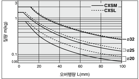
그래프 [9] V=~1000mm/s ~30st
