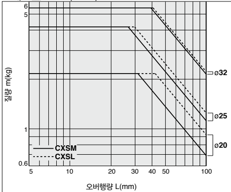
그래프 ⑤ V=1000(mm/s)
