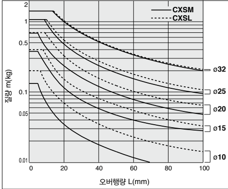
그래프 15 V=400mm/s 초과 ~50st
