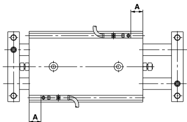
리드선 취출방향 / 안쪽 방향 부착
