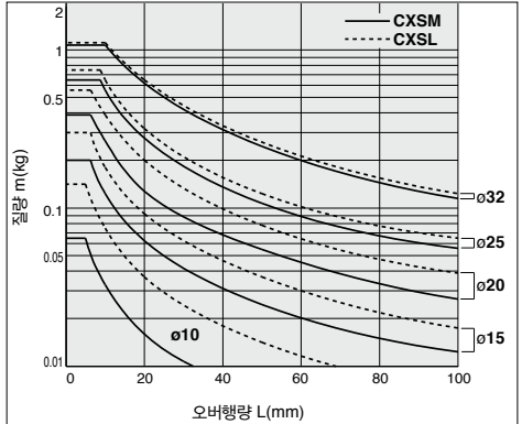
그래프 16 V=400mm/s 초과 ~75st
