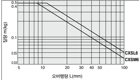
그래프 ① V=100(mm/s)
