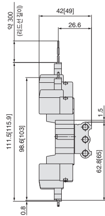
L형 플러그 커넥터(L)
