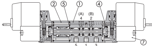
(본 그림은 Closed Center의 경우)
