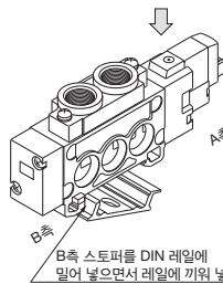
그림1. 밸브 장착 요령
