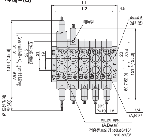
단독 EXH 스페이스서 부착 시의 치수
