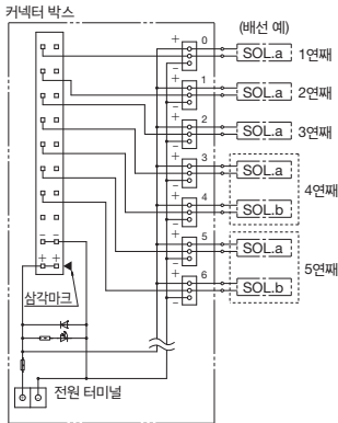
+COM 전기 회로도
