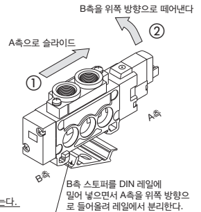
그림2. 밸브 분리 요령
