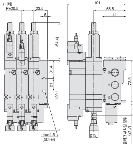
스페이서형 감압 밸브 부착의 경우(게이지 부착)
