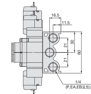
단독 EXH 스페이스 부착 시의 치수
