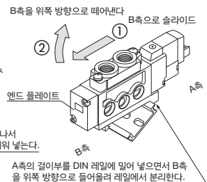
그림2.밸브 분리 요령
