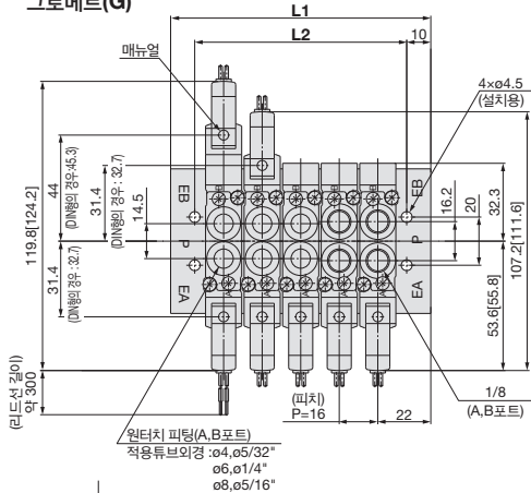
단독 EXH 스페이스 부착 시의 치수
