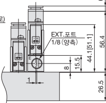
단독 EXH 스페이스 부착 시의 치수
