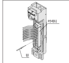
그림4 D서브 커넥터(45F)의 경우
