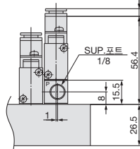
단독 SUP 스페이서 부착 시의 치수 (SUP포트는 싱글 슬레노이드의 엔드 플레이트 축입니다.)
