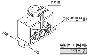
원터치 피팅 배관 (인치 사이즈)
