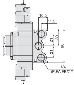
단독 EXH 스페이스서 부착 시의 치수
