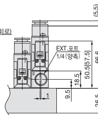
단독 EXH 스페이스서 부착 시의 치수
