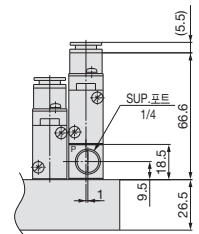
단독 SUP 스페이스서 부착 시의 치수 (SUP 포트는 상글 솔레노이드의 엔드 플레이트 측입니다.)
