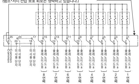
커넥터 결선도[예 : 본 그림의 경우]
