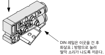
그림1 블록 장착 요령
